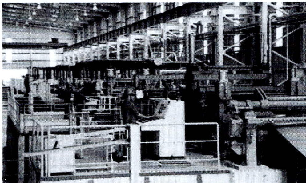
Hình 6: Dây chuyền tẩy rỉ
