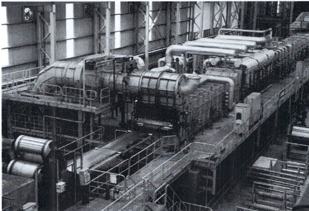
Hình 10: Hệ thống lò ủ NOF của Tôn Đông Á
