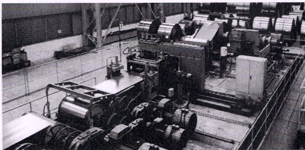
Hình 8: Dây chuyền chia cuộn
