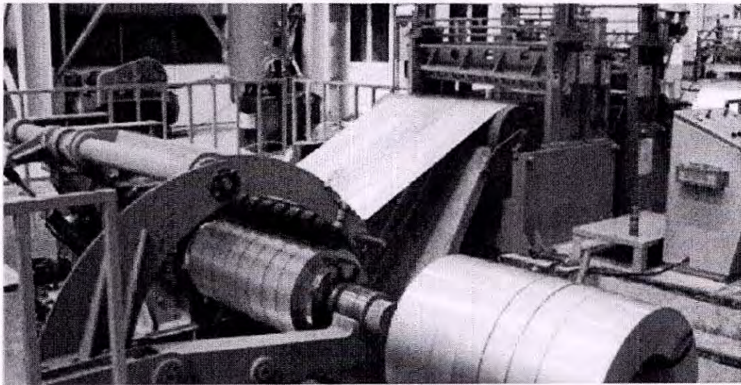
Hình 18: Dây chuyền xả bang của Tôn Đông Á
